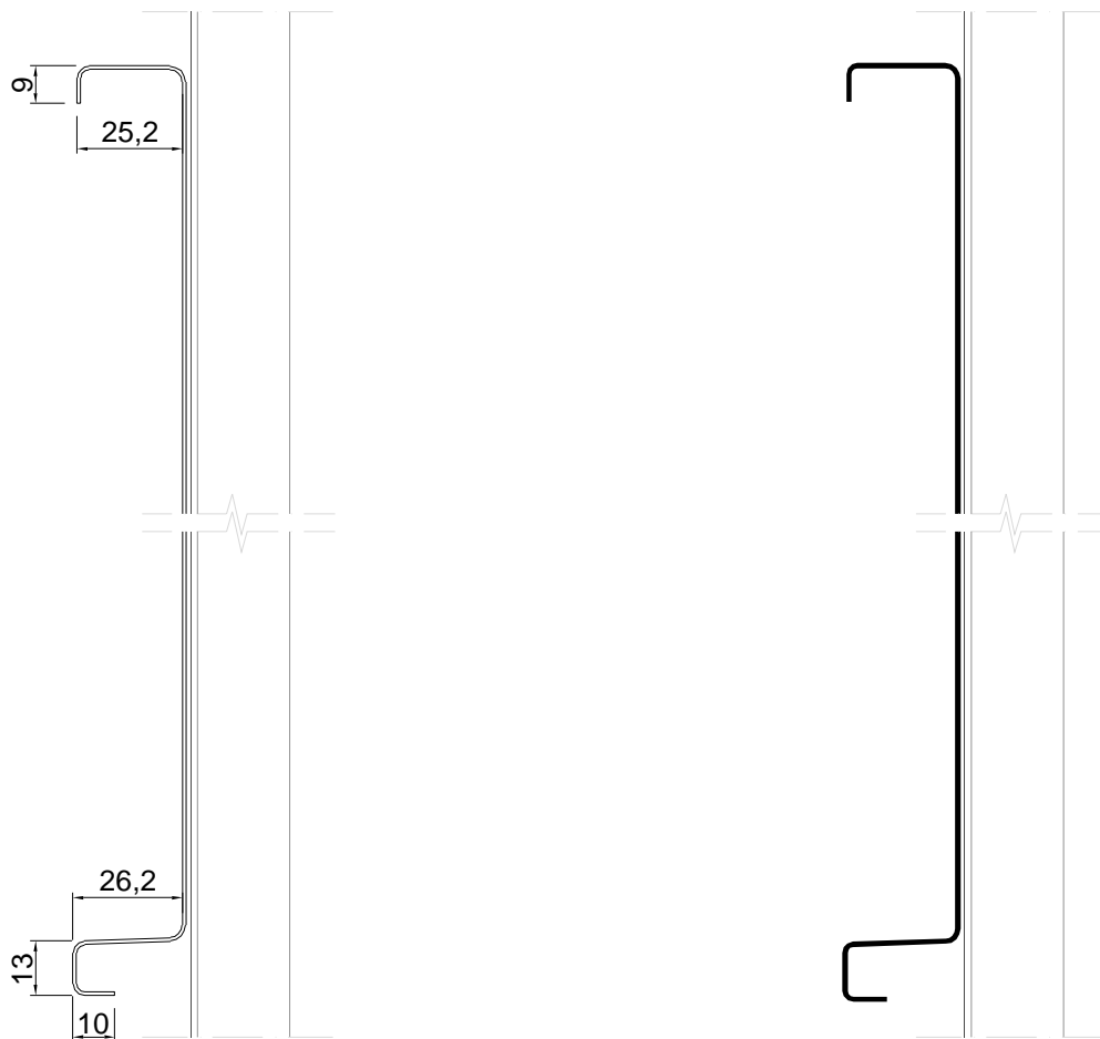
JUNTA ALZADA PERFIL CONFORMADO
