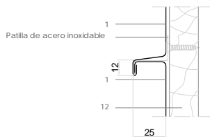
A-A: JUNTA ALZADA EN ÁNGULO SOBRE ENTARIMADO
