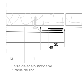
C-C: JUNTA ALZADA EN ÁNGULO SOBRE ENTARIMADO
