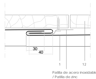
B-B: JUNTA ALZADA EN ÁNGULO SOBRE ENTARIMADO
