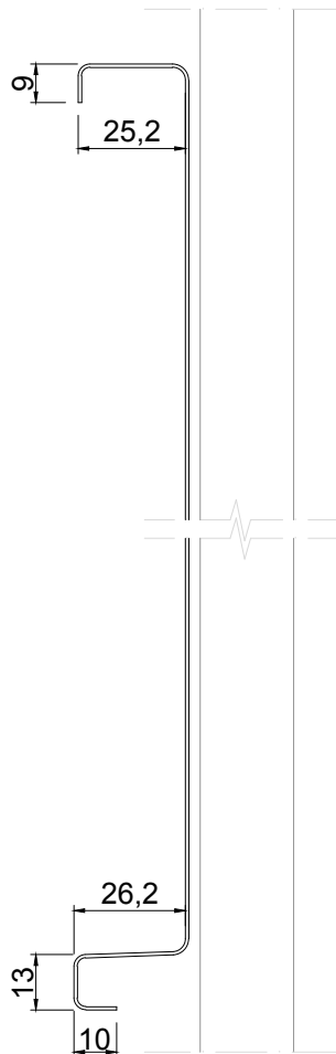
PROFIL DE BAC A JOINT DEBOUT
