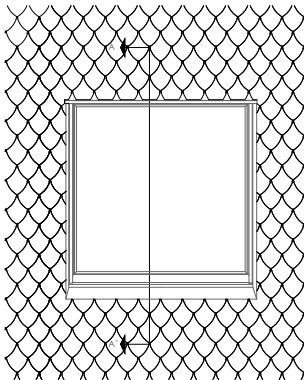
T PF 7.1.01 Vertical window section (Vented sill).
