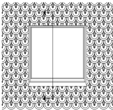
T RF 7.1.01 Vertical window section (Vented sill).
