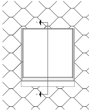
T S 7.1.01 Vertical window section (Vented sill).
