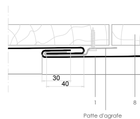
B-B'. COUPE SUR SECTION TRANSVERSALE ENTRE BACS
