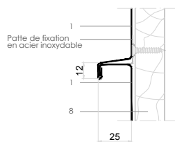
A-A'. COUPE SUR JOINT DEBOUT SIMPLE SERTISSAGE
