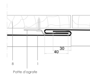
C-C'. COUPE SUR SECTION TRANSVERSALE ENTRE BACS
