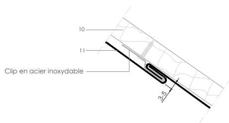
COUPE A-A'
