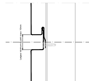
A-A': DETAIL DE JONCTION HORIZONTALE
