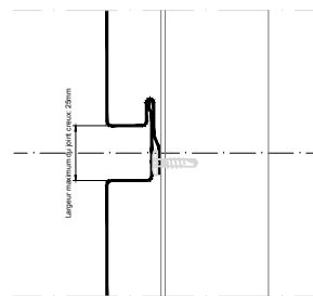
A-A': DETAIL DE JONCTION HORIZONTALE
