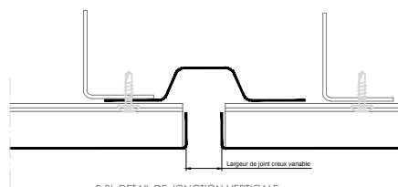
B-B': DETAIL DE JONCTION VERTICALE
