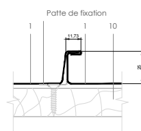
A. JOINT DEBOUT SIMPLE SERTISSAGE
