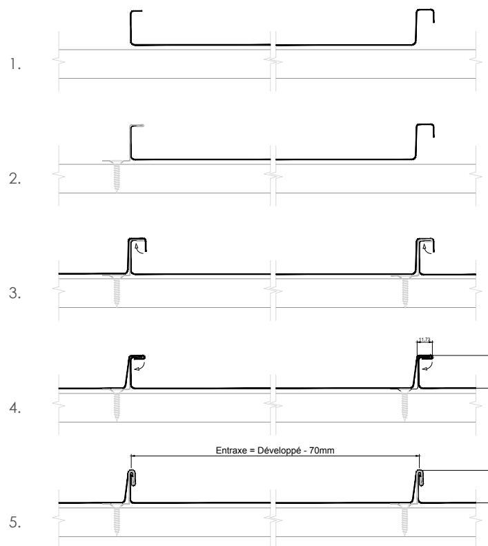
ETAPES DU SERTISSAGE - PROFIL A JOINT DEBOUT
