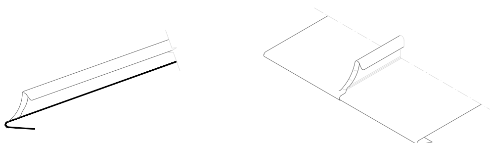
FINITION A L'EGOUT - JOINT A LANGUETTE ETIREE
