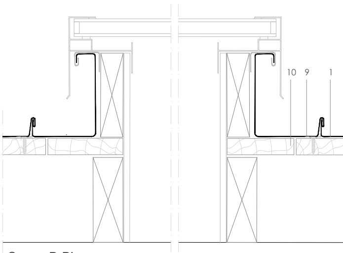
Coupe B-B'
