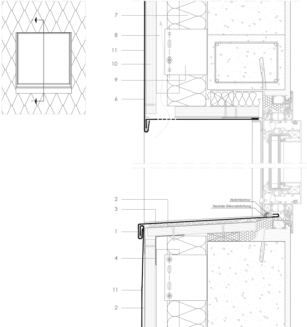
TR 7.2.01 Sección vertical de ventana (alfeizar no ventilado).
