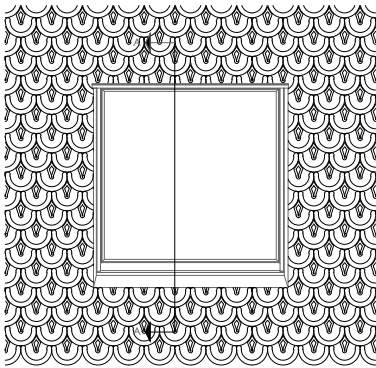
T RF 7.1.01 Vertikaler Fensterdurchschnitt mit Belüftung an der Fensterbank.
