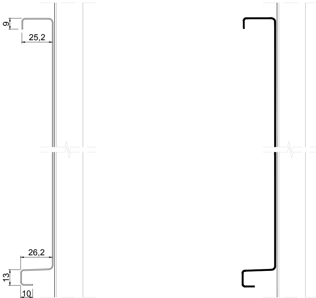
VORPROFILIERTE SCHAR IN WINKELSTEHFALZ
