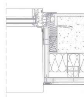
Window jamb
